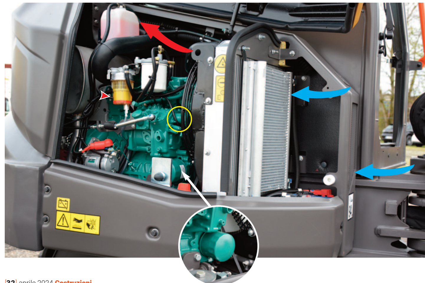
Il motore è sospeso su supporti elastici di notevoli dimensioni per ridurre al massimo le vibrazioni.
